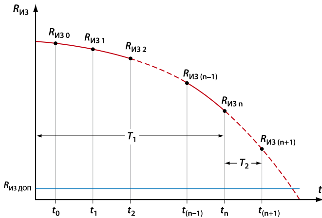
• Рис. 3 Сопротивление изоляции в зависимости от времени
