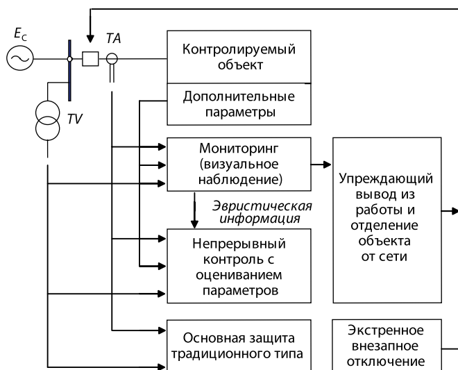
Обобщенная схема функций системы контроля параметров и защиты, обладающей упреждающими свойствами
