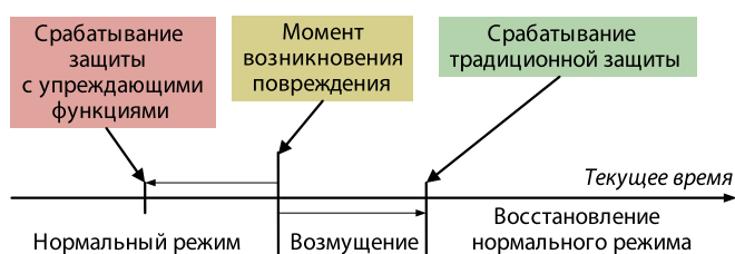
Сравнение действий защиты с упреждающими функциями и традиционной защиты
